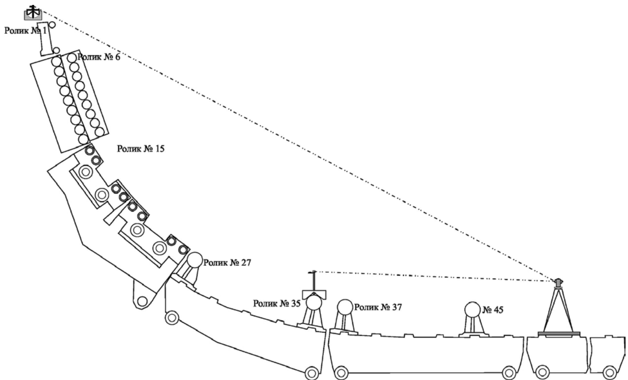
Рис. 12. Схема геодезических измерений МНЛЗ
