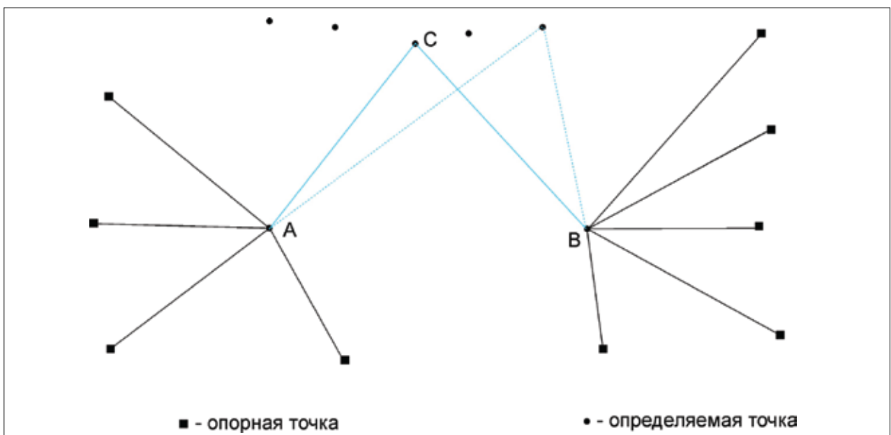
Рис. 4. Схема измерений двумя тахеометрами
